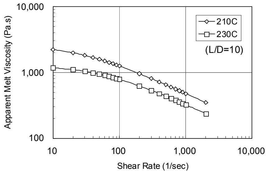
Fig. 1 Melt Viscosity of Soarnol™ D2908
